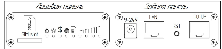
Схема 2 – Расположение индикаторов и портов СИМ-инжектора
