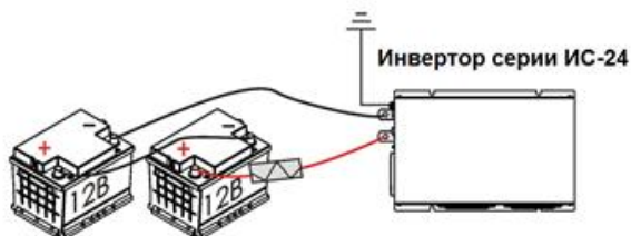
Рисунок 2 Схема подключения инверторов серии ИС
