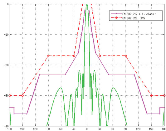
H-Plane Specs
