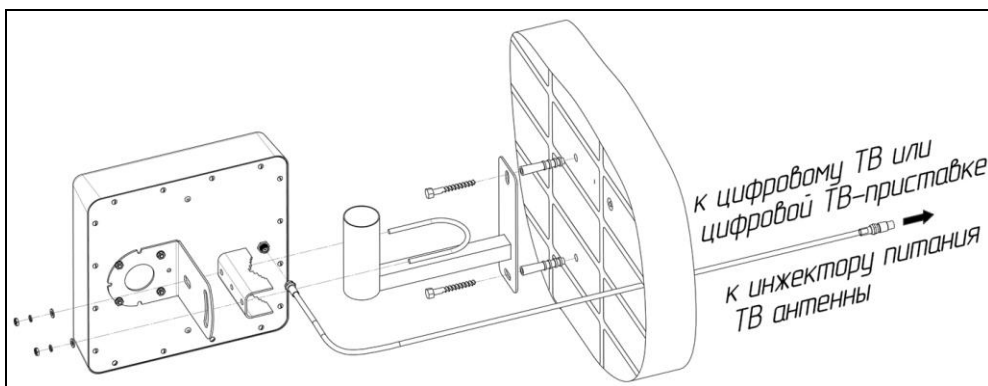
Рисунок 2 – Монтаж антенны на стеновом кронштейне
