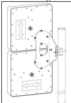
Рисунок 2 – монтаж антенны на мачте
