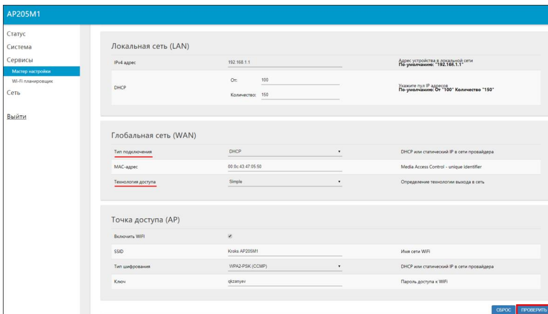
Рисунок 2.1.2 – Настройка подключения по протоколу DHCP-клиент
