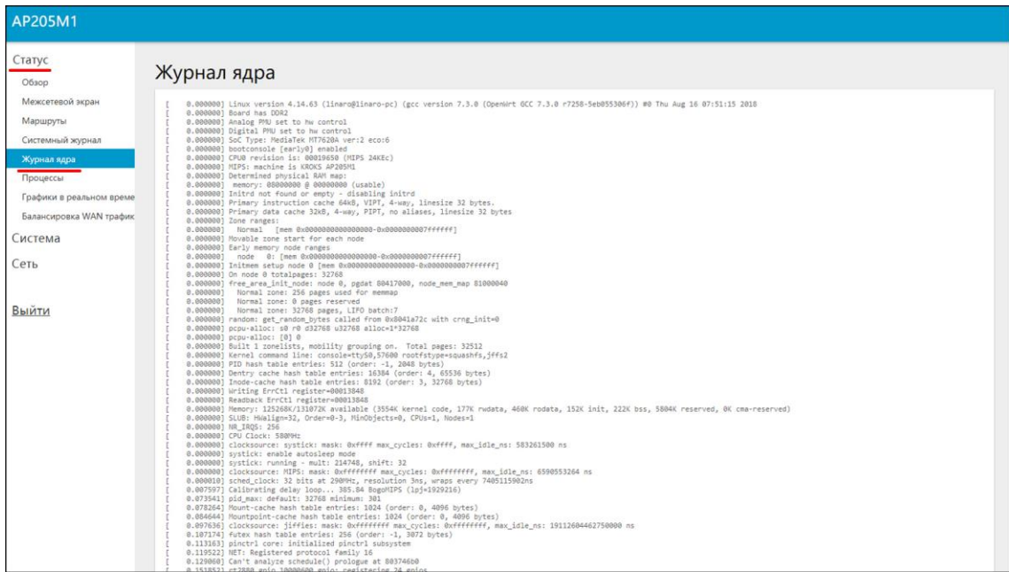
Рисунок 10.4.2 – Журнал ядра
