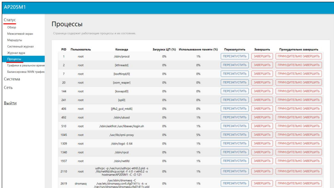
Рисунок 10.5.1 – Диспетчер процессов
