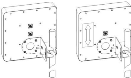
Рисунок 2 – монтаж антенны на мачте
