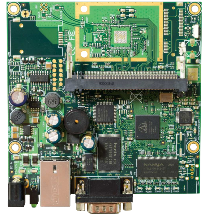
RB411
