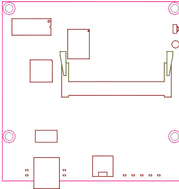
RB411L
