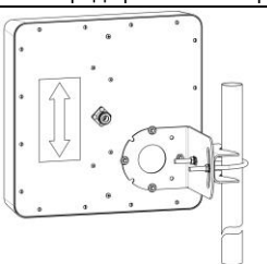
Рисунок 3 – монтаж антенны на мачте
