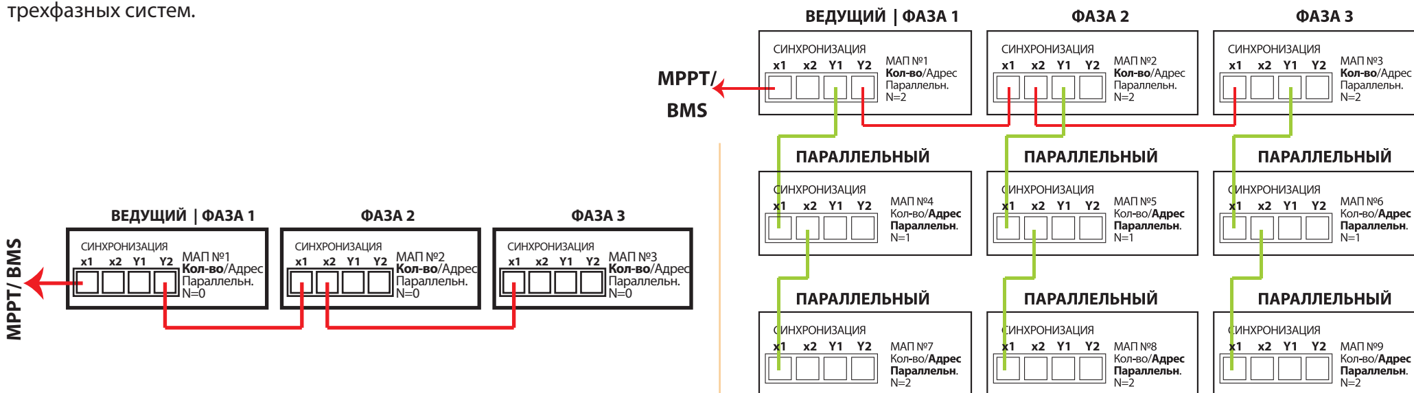
Рис.9 Комбинированная схема трехфазного соединения с параллельным соединением МАП-ов, пример на 9 приборов.
