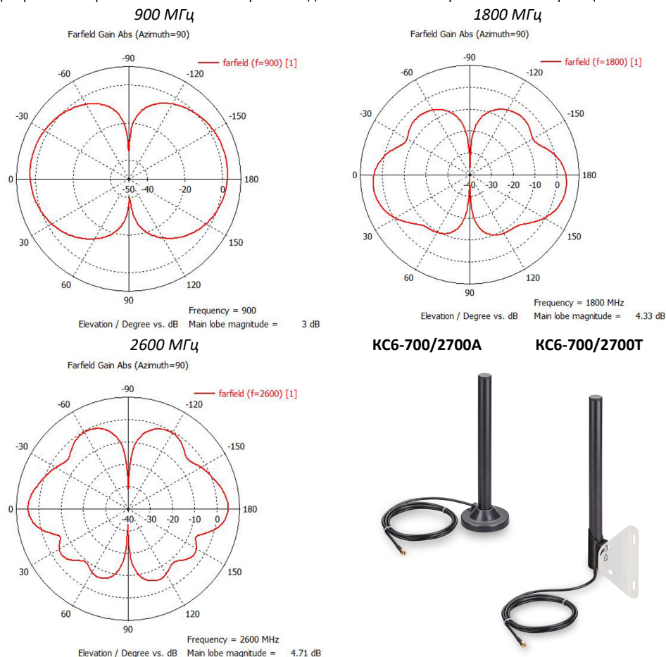
Коэффициент усиления антенны в рабочем диапазоне частот
