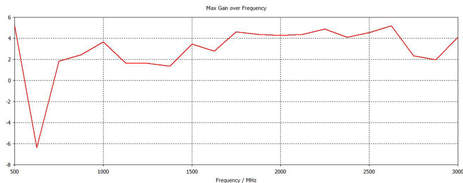
Коэффициент усиления антенны в рабочем диапазоне частот
