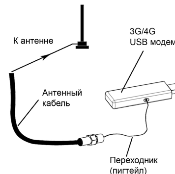
Схема 1 – Подключение антенны к USB модему
