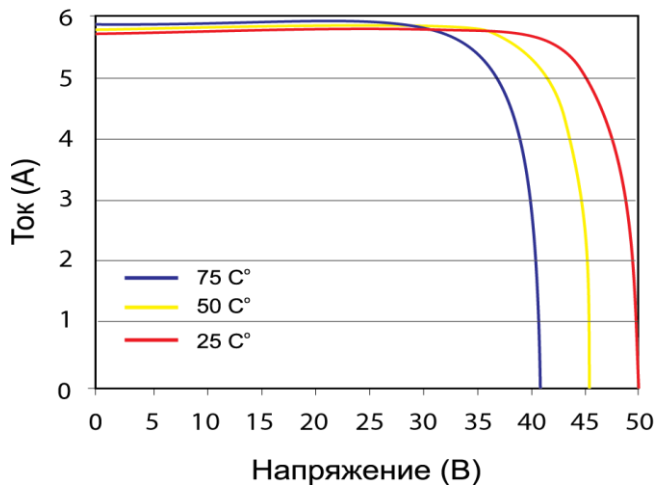
Зависимость электрических параметров от температуры окружающей среды
