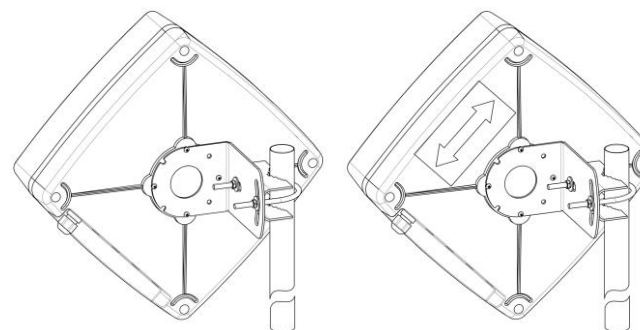
Рисунок 4 – X-поляризация
